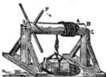
Torno.—B-P, potencia; A-B-C, apoyo; F, resistencia
